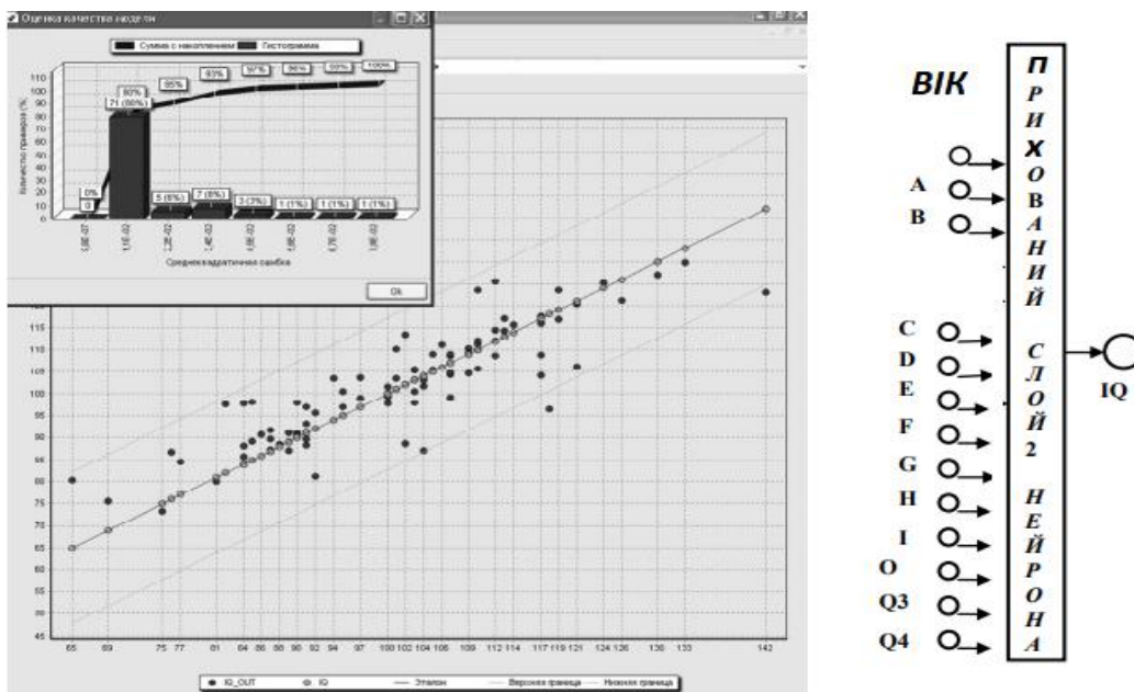
Рисунок 1. Структура ІНС
